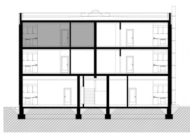
SCHEMA UMÍSTĚNÍ BYTU, ŘEZ
