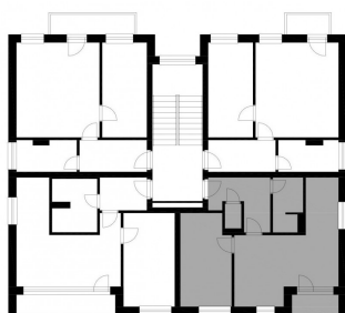
SCHÉMA UMÍSTĚNÍ BYTU, PŮDORYS 2NP
