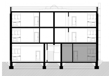
SCHÉMA UMÍSTĚNÍ BYTU, ŘEZ
