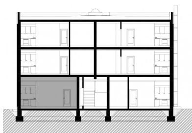
SCHÉMA UMÍSTĚNÍ BYTU, ŘEZ
